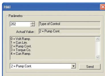
Дистанционный интерфейс "человек-машина" для изменения параметров
