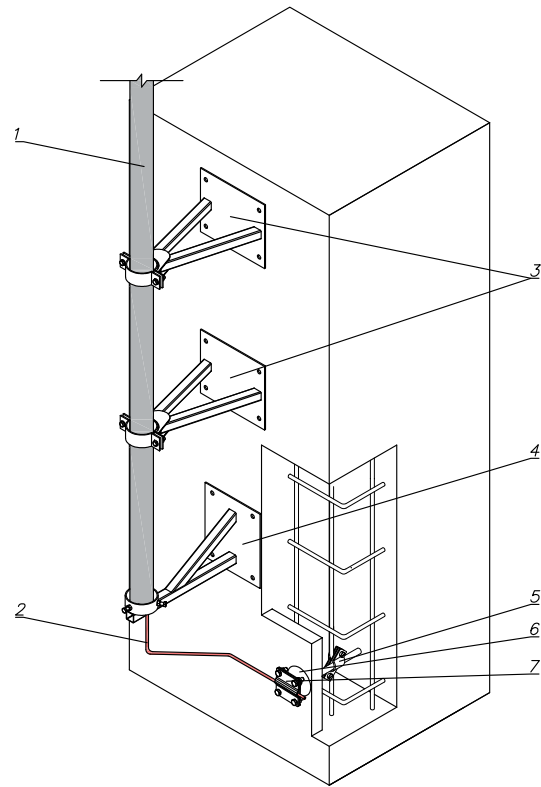
Узел заземления
