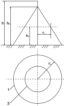
Зоны защиты одиночного стержневого молниеприемника
