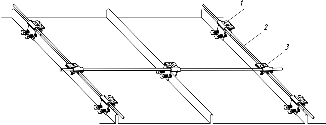
Узел фиксации прутка на фальцевой кровле
