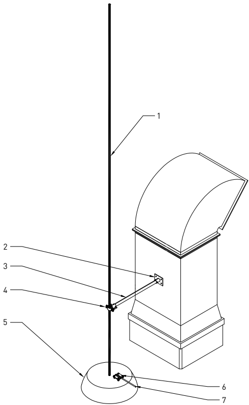
Система молниезащиты вентиляционной шахты
