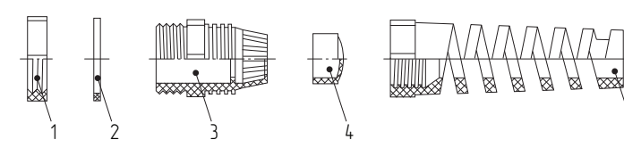
1 – Гайка крепежная (S 1 ) 2 – Кольца уплотнительные 3 – Корпус кабельного ввода 4 – Уплотнитель кабеля 5 – Гайка накидная-ввод спиральный (S)
